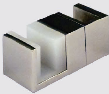
Guía inferior y anclaje vidrio fijo Inox brillo Vidrio 8-10 mm (recom: 8 mm)
