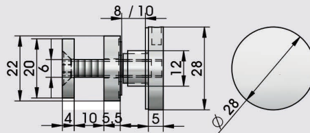
Anclaje vidrio fijo-carril Inox brillo Vidrio: 8-10 mm (recom: 8 mm)
