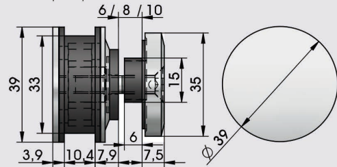
Cojinete Inox brillo Peso max. 40 kg/puerta Vidrio: 6-8-10 mm (recom: 8 mm)
