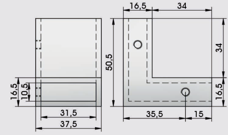
Conexión 90° carril-vidrio fijo Inox brillo Vidrio: 8-10 mm (recom: 8 mm)
