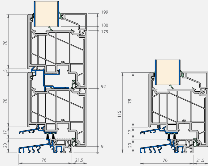
Secciones verticales
