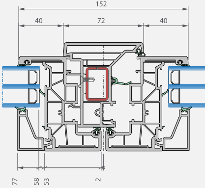
Sección horizontal
