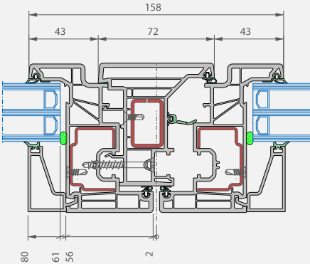
Sección horizontal
