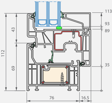
Sección vertical
