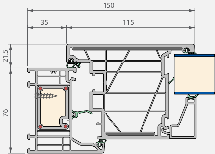
Sección horizontal
