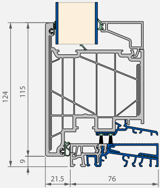
Sección vertical
